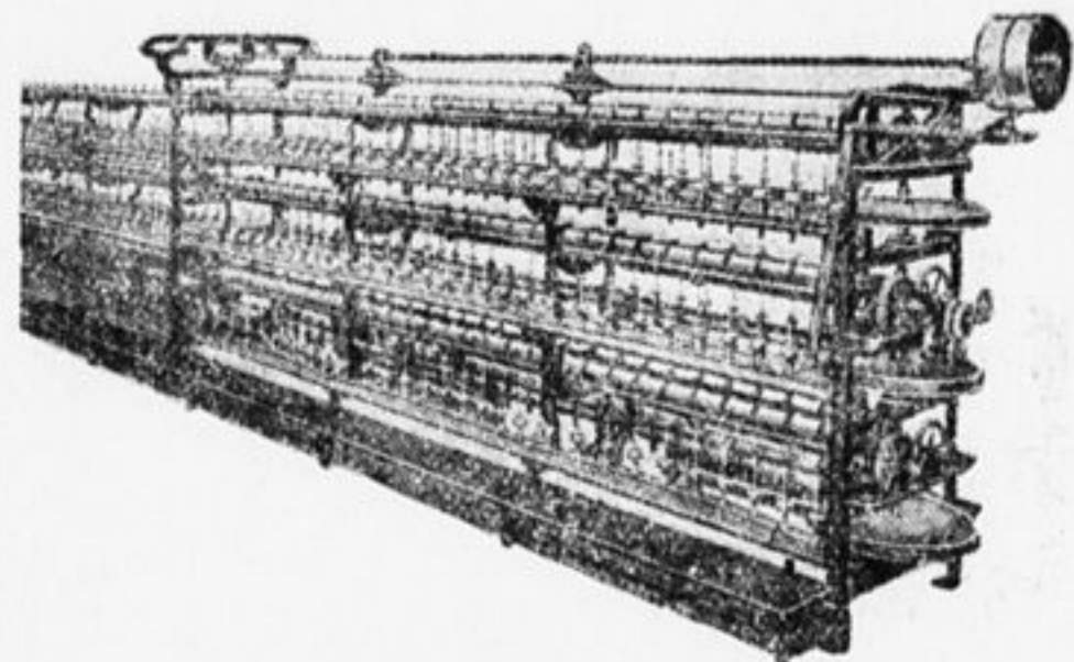
Шелко-крутильная машина.
